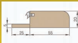
Próg z twardego drewna liściastego szer. 55 mm, lakierowany bezbarwny.
