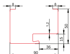
Ościeznica stalowa z uszczelką FD-25/21B
