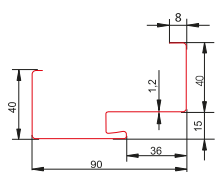
Ościeznica stalowa z uszczelką FD-25/21C
