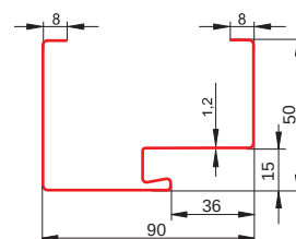
Ościeżnica stalowa z uszczelką do drzwi stalowych zewnętrznych 55, 55 LUX FD-25/21B-55
