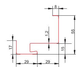
Ościeżnica stalowa z uszczelką do drzwi stalowych technicznych 40 FD-21/N
