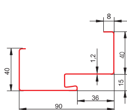
Ościeżnica stalowa z uszczelką do drzwi stalowych zewnętrznych 55, 55 LUX FD-25/21C-55
