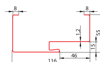
Ościeżnica stalowa z uszczelką do drzwi stalowych zewnętrznych 72 LUX FD-25/21B-72
