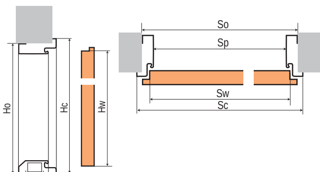
Rys. nr 1 Osadzenie ościeżnicy narożnej na mur
