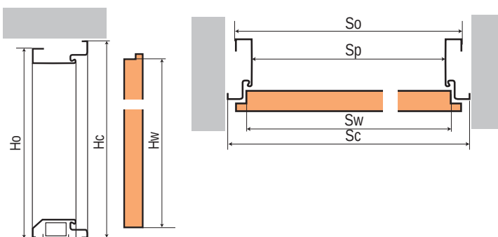
Rys. nr 2 Osadzenie ościeżnicy wewnątrz muru
