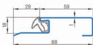
Próg stalowy.
