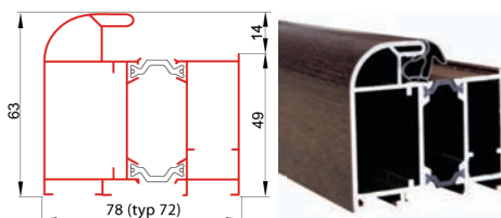
Ciepła ościeżnica aluminiowa z uszczelką do drzwi stalowych zewnętrznych 72 LUX, 72 LUX TERMO, 85 LUX TERMO PLUS
