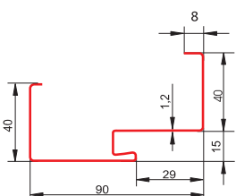
Ościeżnica stalowa z uszczelką do drzwi stalowych technicznych 40 FD-25/21C-40
