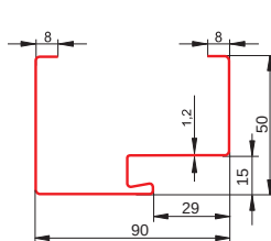
Ościeżnica stalowa z uszczelką do drzwi stalowych technicznych 40 FD-25/21B-40
