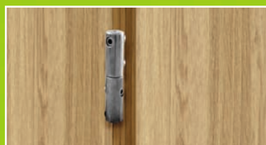
Regulowane trzy zawiasy 2-czopowe (drzwi przylgowe).
