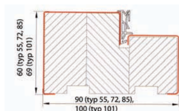
Ciepła ościeżnica stalowo-drewniana z uszczelką do drzwi stalowych zewnętrznych 55, 55 LUX, 72 LUX, 72 LUX TERMO, 85 LUX TERMO PLUS, 101 LUX TERMO PLUS
